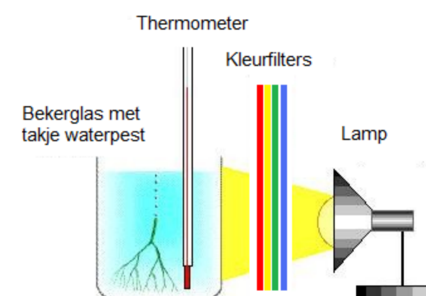
Opstelling herhalingspracticum
